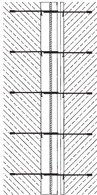
Bild 15: Regeldetail Schlaufenüberlappung
