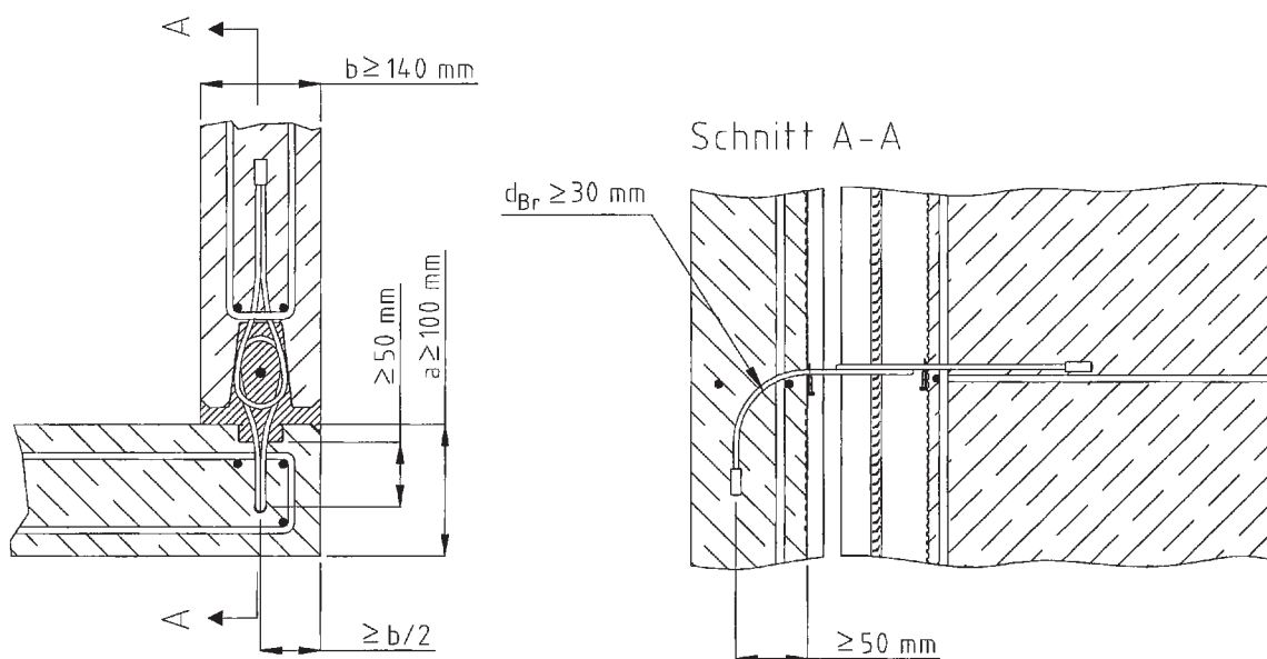
Bild 8: Wand - Wand – Eckverbindung - Detail bei abgewinkelter Seilschleufe
