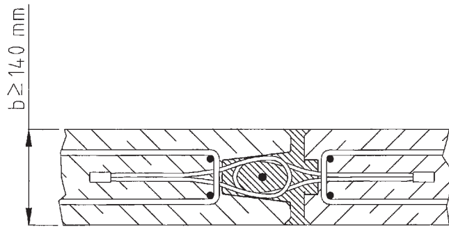
Bild 5: Wand - Wandverbindung
