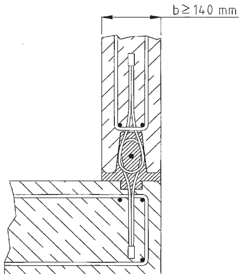
Bild 7: Wand - Wand – Eckverbindung - Regeldetail
