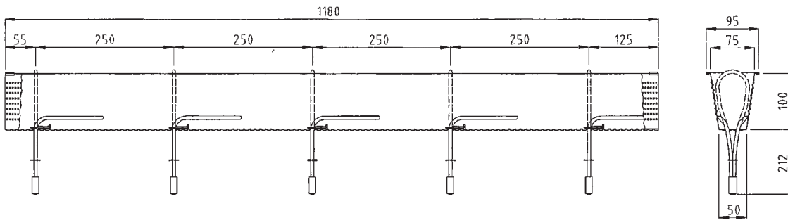
Bild 1: VS®-Schiene TZ100 (Längs- und Querschnitt)
