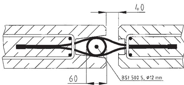
Bild 14: Maximale Fugenbreite
