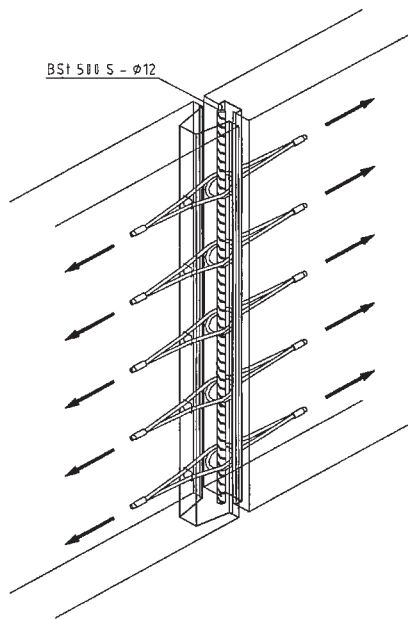
Bild 17: Zugbeanspruchung in Schlaufenlängsrichtung
