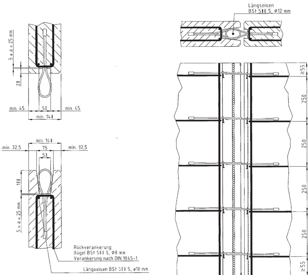
Bild 11: Vergussnut, Bewehrung
