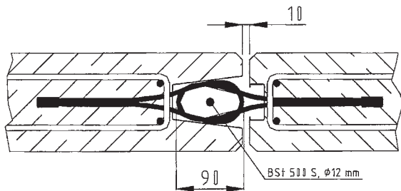
Bild 13: Minimale Fugenbreite
