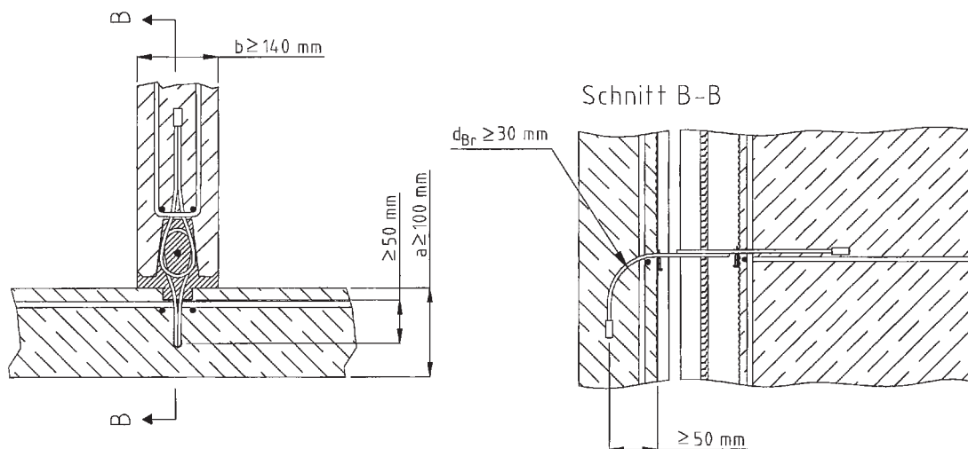
Bild 10: Wand - Wand – T-Verbindung - Detail bei abgewinkelter Seilschleufe
