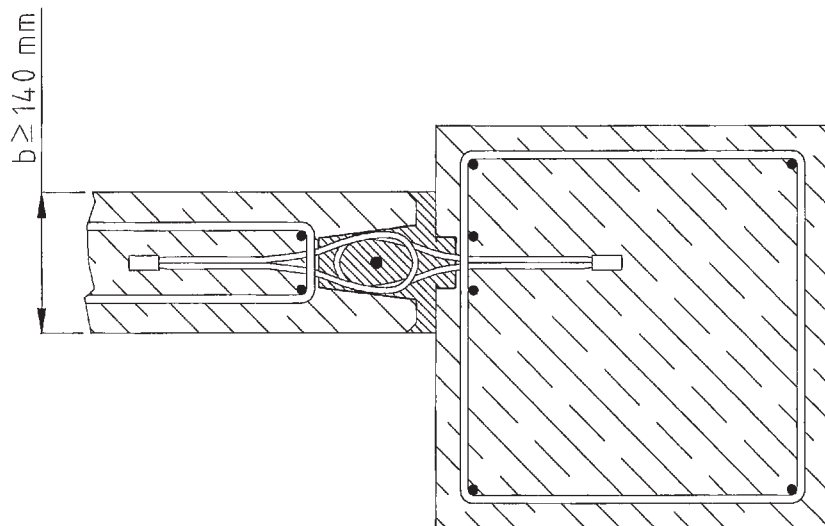
Bild 6: Stützen - Wandverbindung
