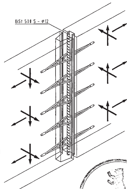
Bild 20: Kombinierte Beanspruchung
