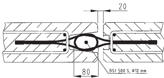
Bild 12: Regelfall Fuge
