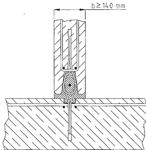
Bild 9: Wand - Wand – T-Verbindung - Regeldetail
