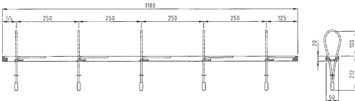
Bild 3: VS®-Leiste TZ100 (Längs- und Querschnitt)
