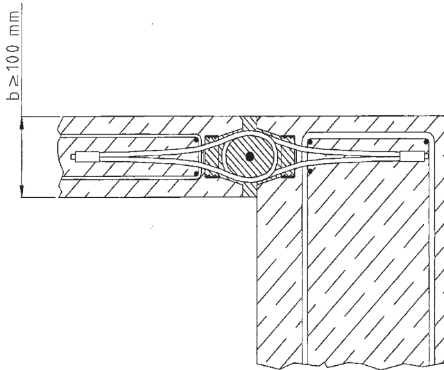
Bild 5: Wand – Wand – Eckverbindung - Regeldetail
