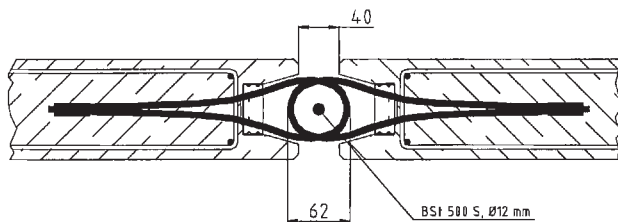
Bild 12: Maximale Fuge
