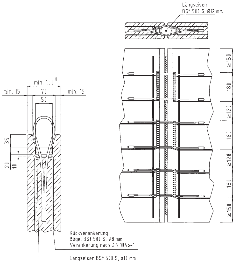
Bild 9: Vergussnut, Bewehrung
