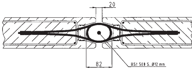
Bild 10: Regelfall Fuge
