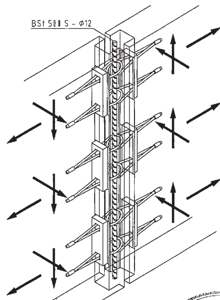
Bild 18: Kombinierte Beanspruchung
