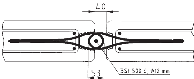
Bild 14: Maximale Fugenbreite
