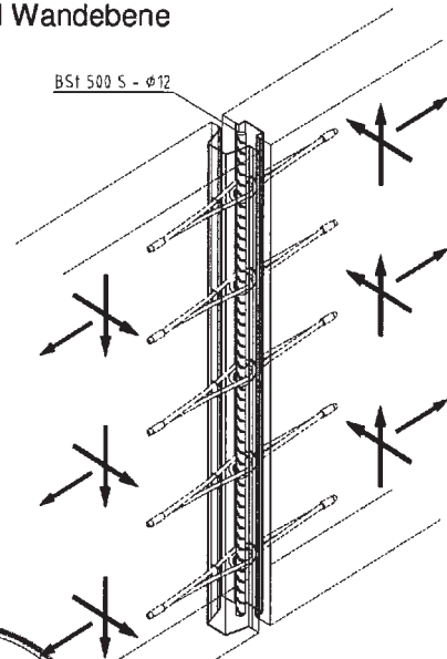
Bild 20: Kombinierte Beanspruchung
