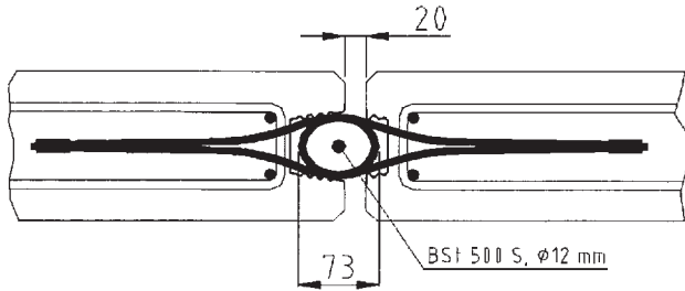
Bild 12: Regeldetail Fuge
