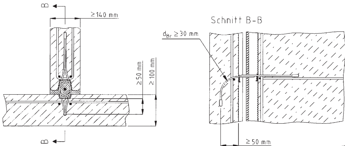
Bild 10: Wand - Wand – T-Verbindung - Detail bei abgewinkelter Seilschleufe
