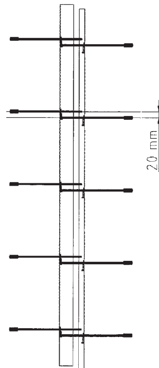
Bild 16: Maximale vertikale Fehllage: 20 mm
