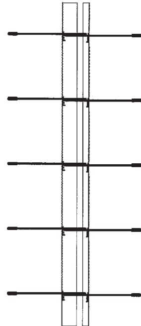
Bild 15: Regeldetail Schlaufenüberlappung
