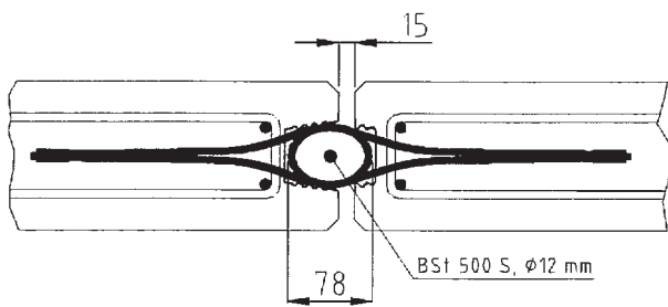
Bild 13: Minimale Fugenbreite
